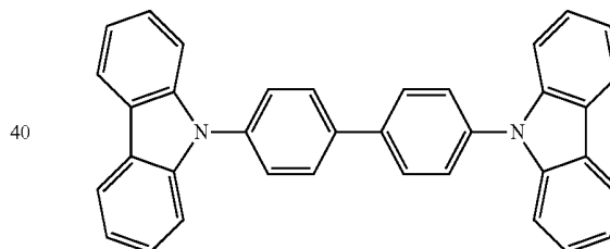
CBP
